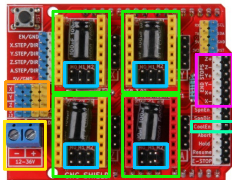
Motoranschlüsse Versorgung 12-36V Treibersteckplätze Microstepping-Jumper Endstop-Anschlüsse Mosfet-Anschluss
